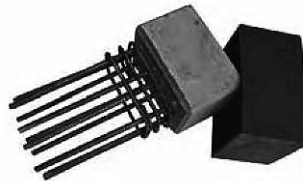
Typ/Type TSB-BT Schall-Isobox/Boîte insonorisante Füllkörper/Remplissage Beton-Tragelement/Élément porteur
